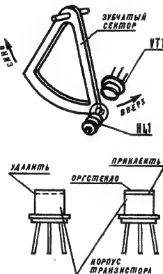
Рис. 3 Конструкция фототранзистора
