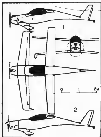
Рис. 4. Современные легкомоторные тандемы. 1. «Кавик» Берта Рутана. 2. А-8 Юрия Яковлева, СССР, СЛА-84.
