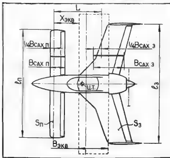
Рис. 4. Схема центровки самолета тандемной компоновки.
