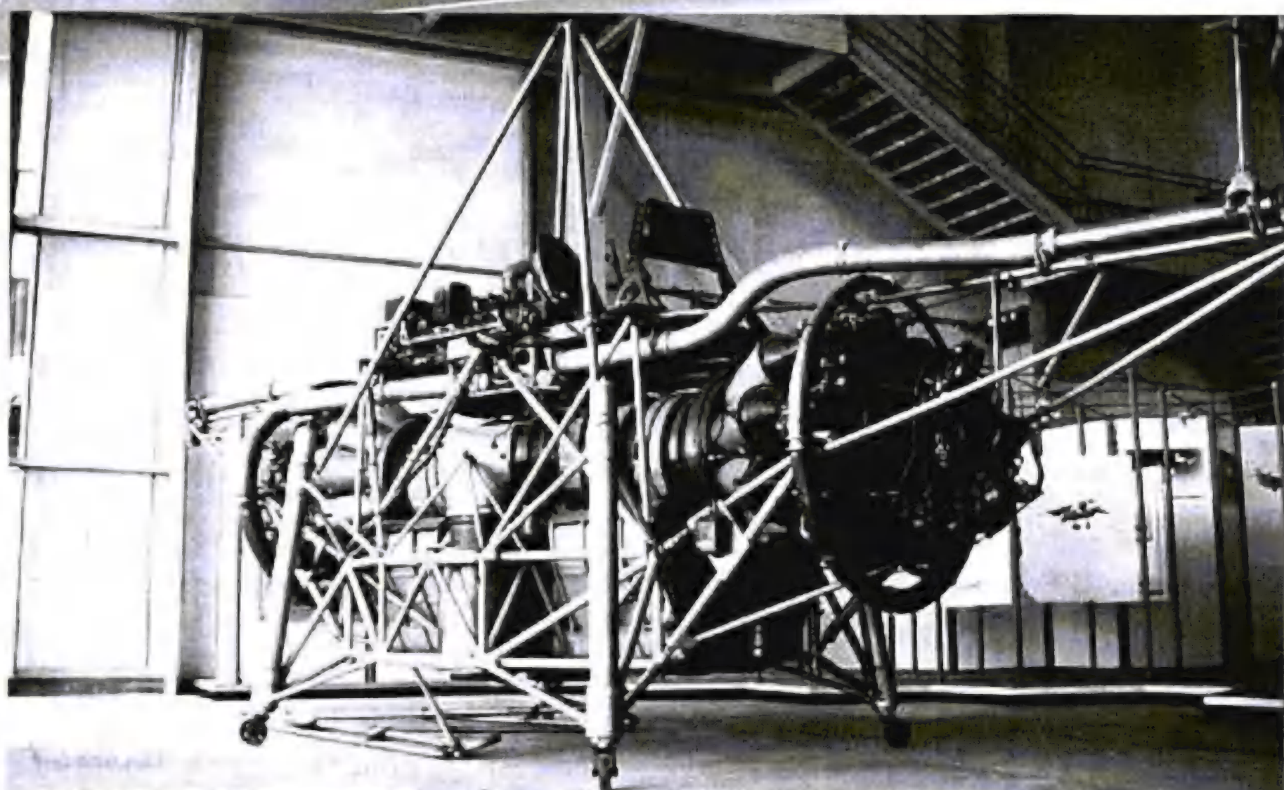
Летающий стенд TMR – «Летающая кровать»
