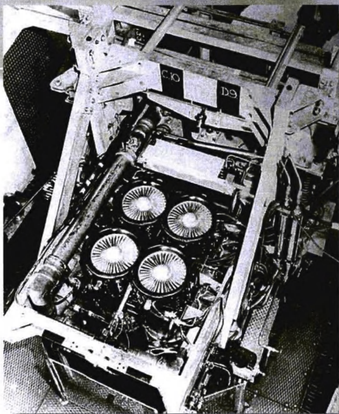
Подъемные двигатели RB-108
