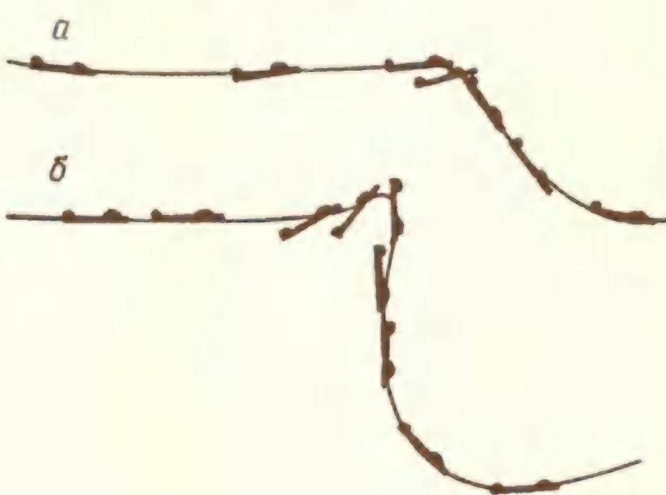
Рис. 1. Срыв планера: а — статический, б — динамический.
