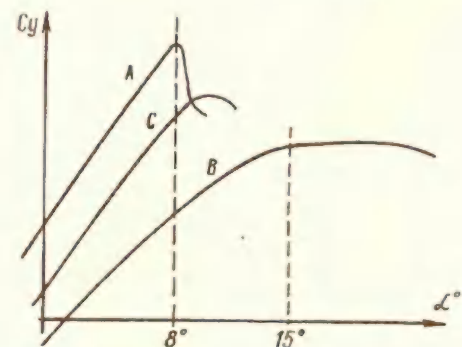
Рис. 2. Зависимость коэффициента подъемной силы от угла атаки при различных положениях закрылков: А — закрылки вниз (+10°), В — закрылки вверх (-10°), С — закрылки нейтрально (0°).
