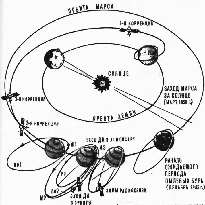
Баллистическая схема экспедиции по проекту Марс-94. (Литерами ПО обозначены переходные, РО — рабочие орбиты искусственного спутника Марса.)
